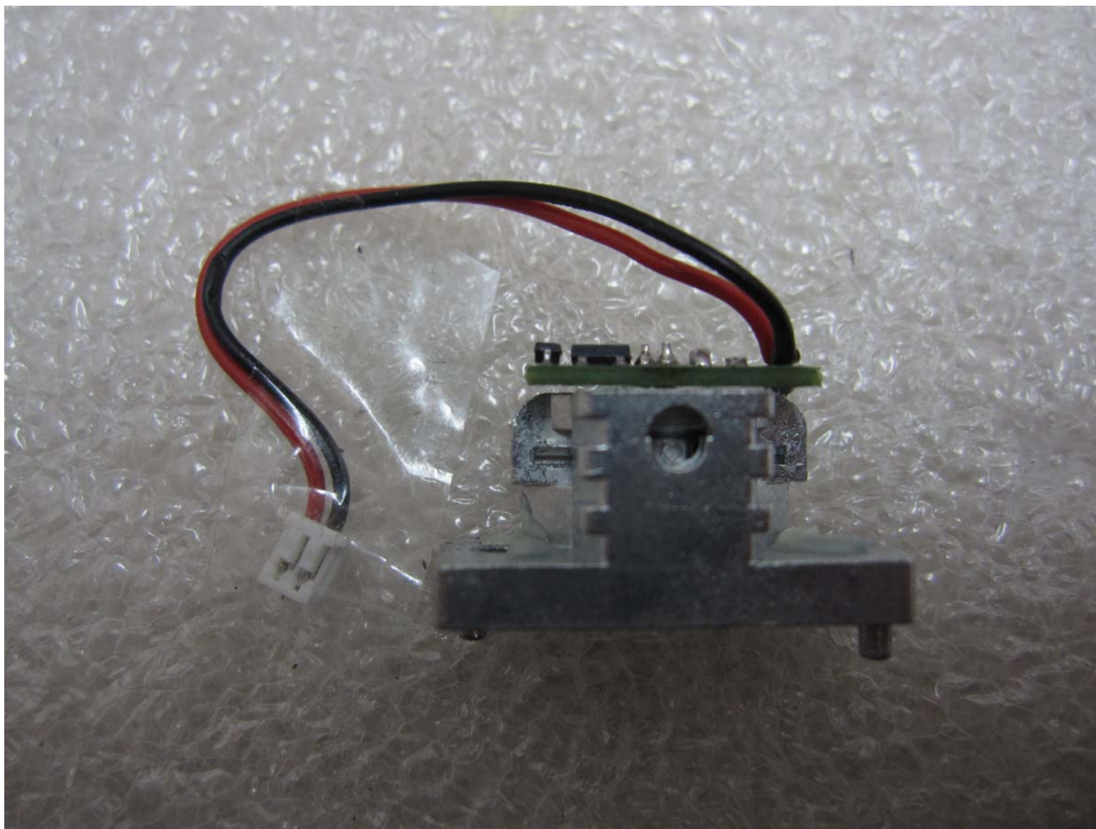
Magic Cube_IR Light Source Module Rear
