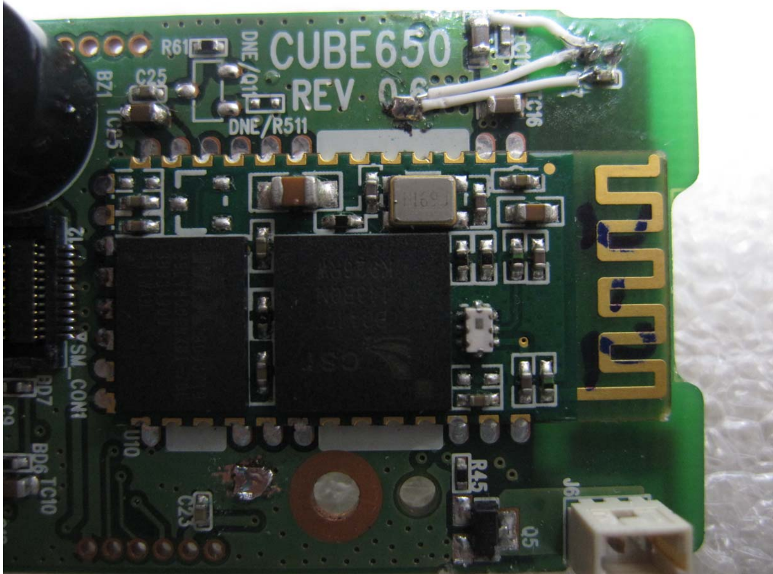
Magic Cube_RF Module
